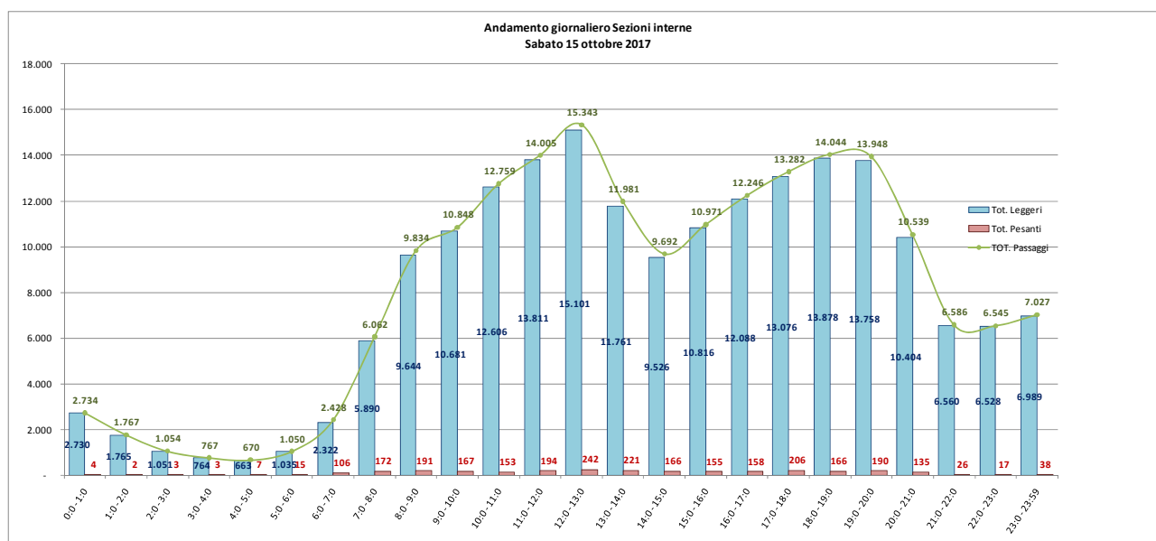
Fig .5.17 – andamento giornaliero (sabato) dei flussi di traffico sul totale delle sezioni interne
