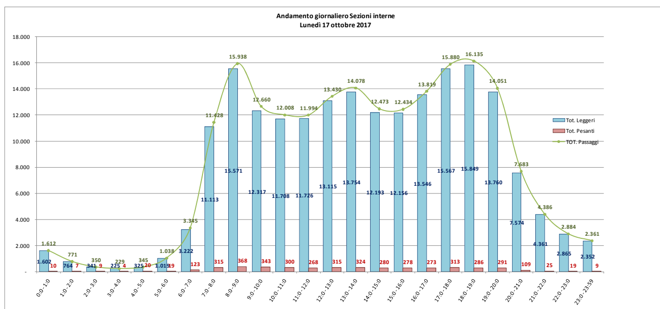
Fig .5.12 – andamento giornaliero (lunedì) dei flussi di traffico sul totale delle sezioni interne
