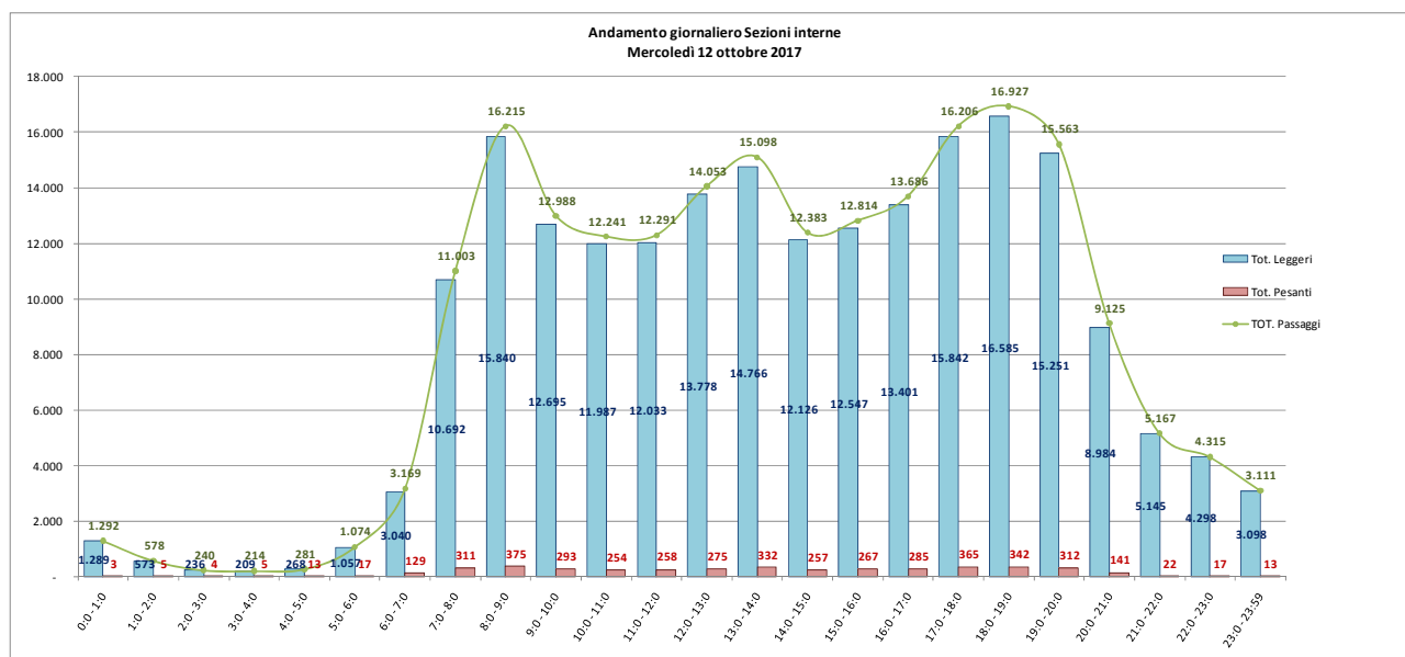
Fig .5.14 – andamento giornaliero (mercoledì) dei flussi di traffico sul totale delle sezioni interne
