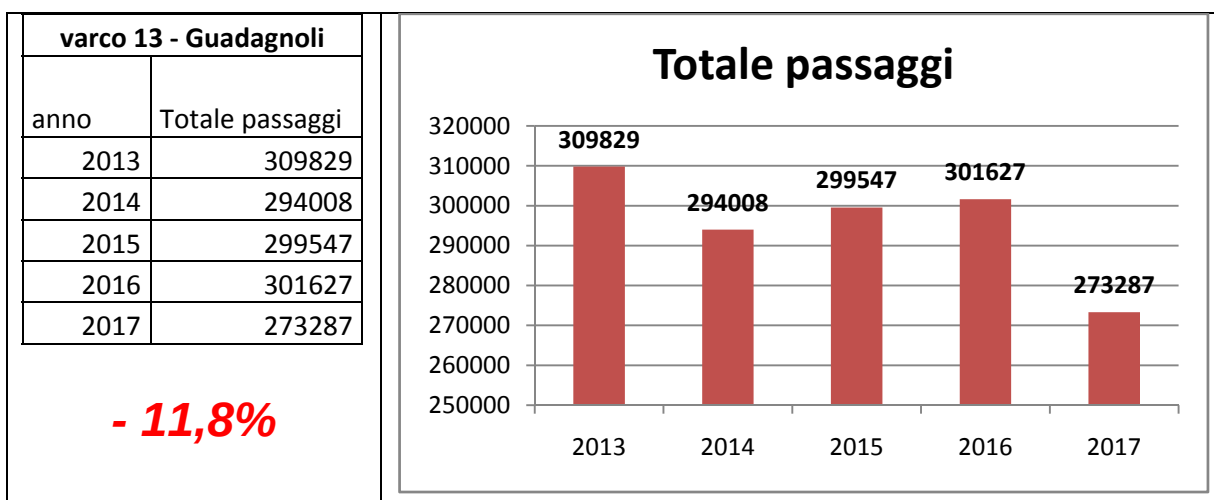
Fig. 5.29 – Serie dati storica flussi di traffico varco di via Guadagnoli
