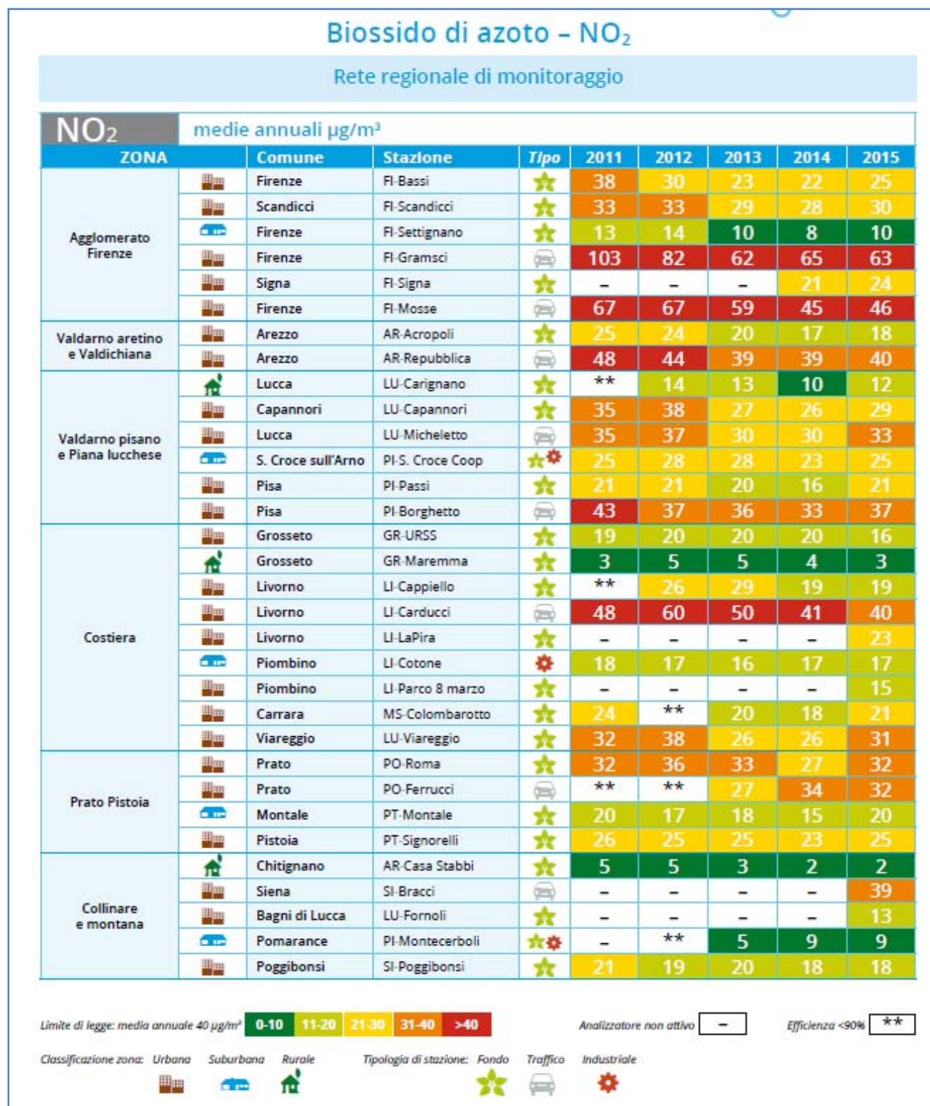
Fig. 3.14 – Biossido di azoto – medie annuali
