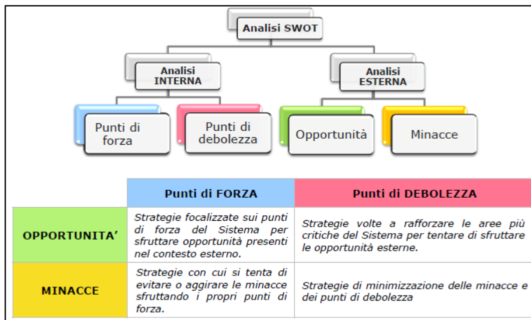
Fig. 6.2 – Analisi SWOT
