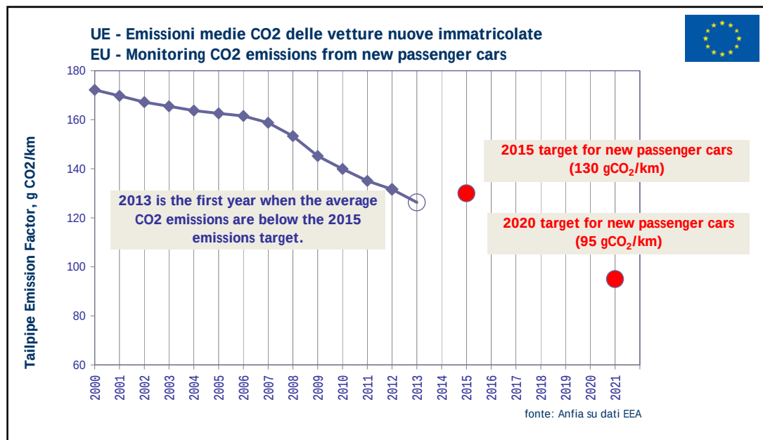
Figura 3.21 – Emissioni medie CO 2 delle autovetture per anno di immatricolazione
