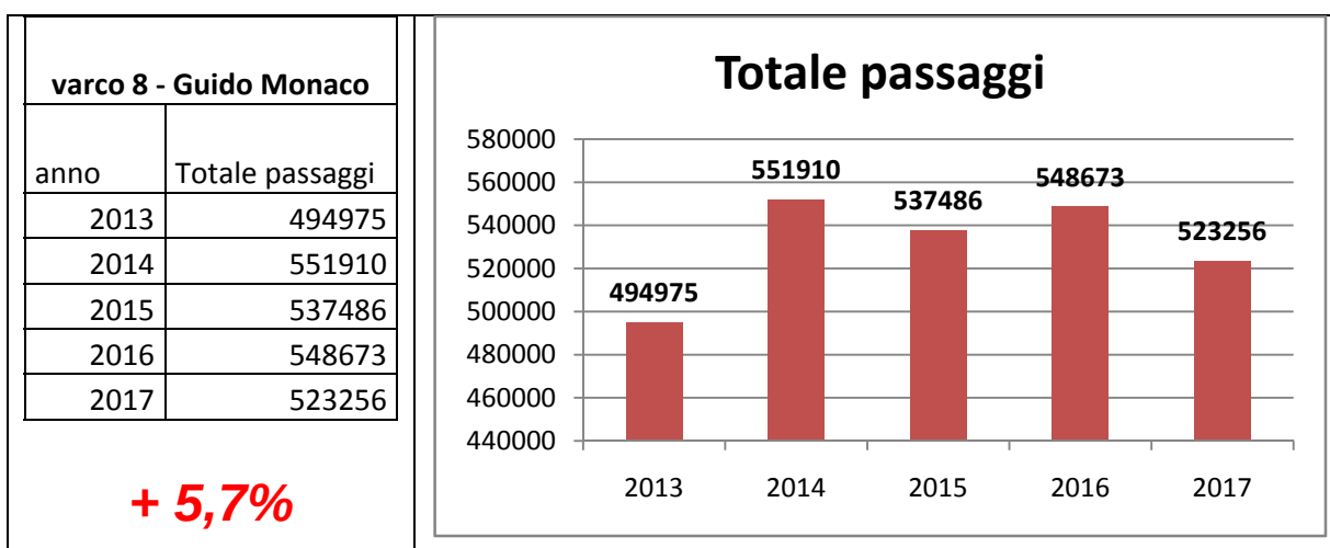
Fig. 5.26 – Serie dati storica flussi di traffico varco di via G. Monaco
