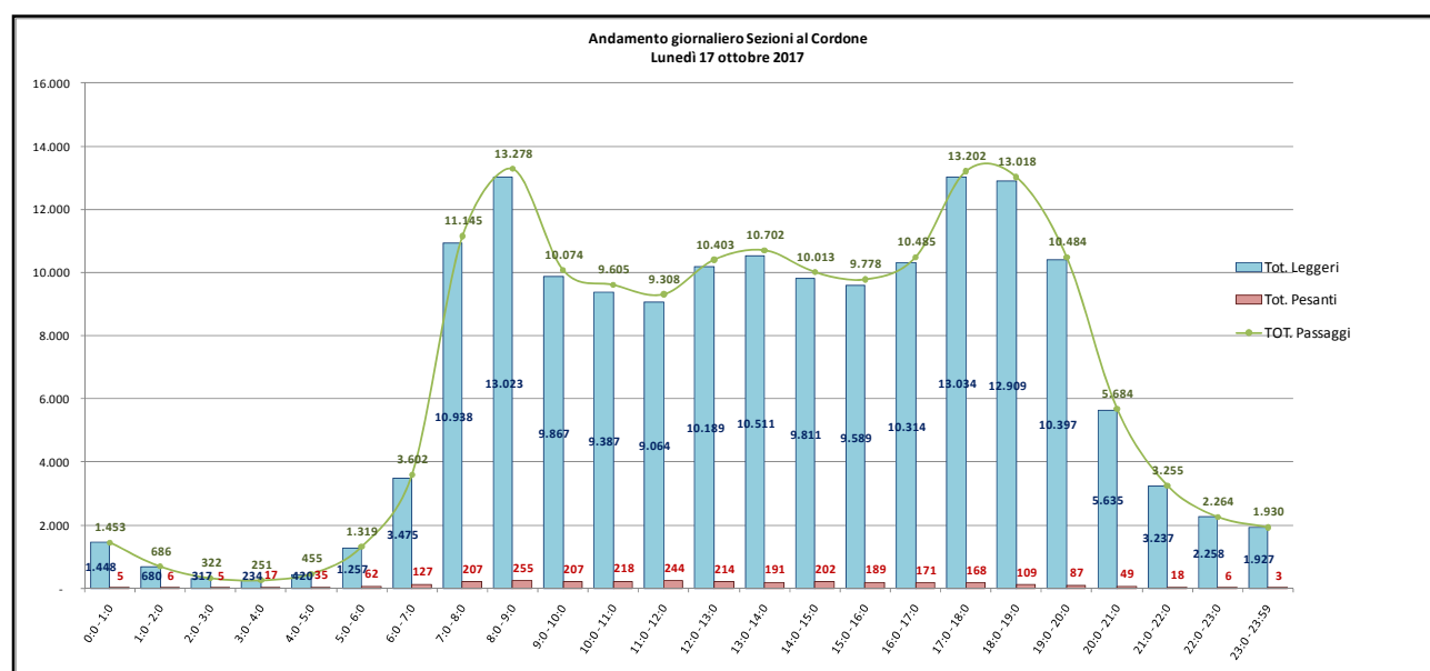
Fig. 5.2 – andamento giornaliero ( lunedì) dei flussi di traffico sul totale delle sezioni “al cordone”
