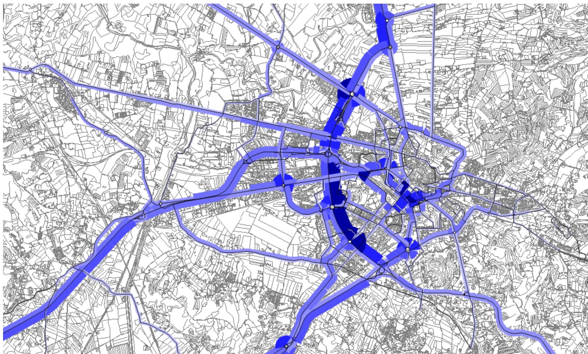
Fig. 10.1 – Flussogramma della rete urbana di Arezzo (ora di punta 7:45-8:45)
