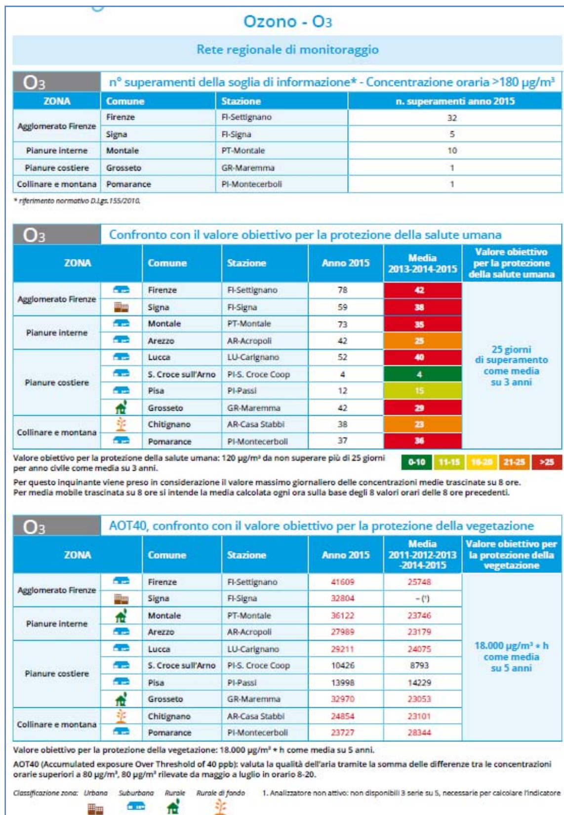
Fig. 3.19 – Ozono
