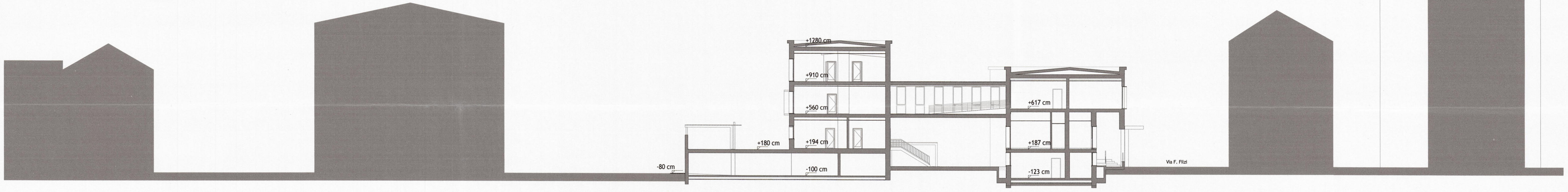
SEZIONE AMBIENTALE A-A Scala 1:200
